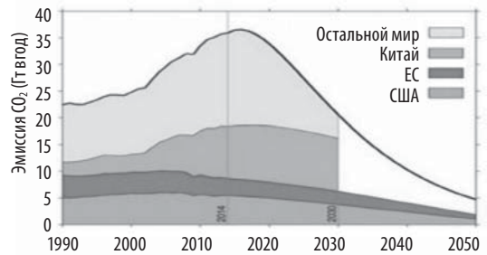
Рисунок 8. Выбросы CO 2 в последние десятилетия в разных регионах Земли
