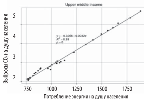
Рисунок 19. Корреляции между средним значением потребления энергии на душу населения за год (кг в нефтяном эквиваленте) и средним значением выбросов CO 2 на душу населения в год (т) по странам с различным уровнем доходов (по базе данных World Bank, 1978–2011 гг.). Диаграмма рассеивания с наложенной линией регрессии
