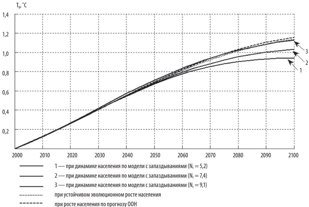
Рисунок 16. Отклонения средней глобальной температуры у поверхности Земли в XXI в. от значения в 2000 г.
