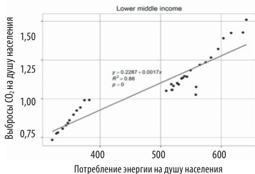
Рисунок 19. Корреляции между средним значением потребления энергии на душу населения за год (кг в нефтяном эквиваленте) и средним значением выбросов CO 2 на душу населения в год (т) по странам с различным уровнем доходов (по базе данных World Bank, 1978–2011 гг.). Диаграмма рассеивания с наложенной линией регрессии
