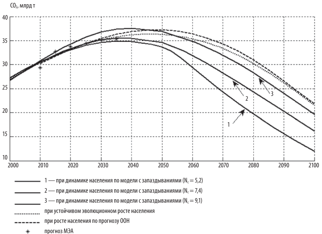
Рисунок 12. Динамика промышленных выбросов CO 2 в XXI в., млрд т
