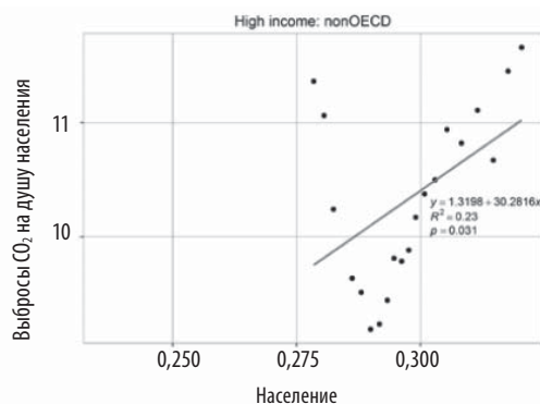
Рисунок 21. Корреляции между средним значением численности населения (млрд человек) и средним значением выбросов CO 2 на душу населения в год (т) по странам с различным уровнем доходов (по базе данных World Bank, 1978–2011 гг.). Диаграмма рассеивания с наложенной линией регрессии
