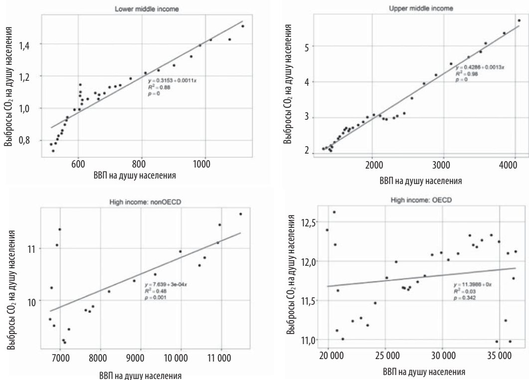
Рисунок 20. Корреляции между средним значением ВВП на душу населения (долл.) и средним значением выбросов CO_2 на душу населения в год (т) по странам с различным уровнем доходов (по базе данных World Bank, 1978–2011 гг.). Диаграмма рассеивания с наложенной линией регрессии
