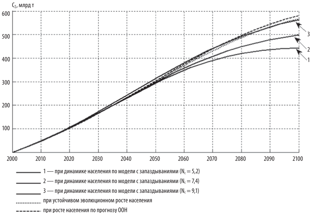
Рисунок 14. Динамика накопления углерода в атмосфере в XXI в.
