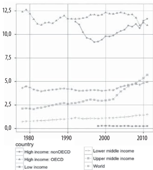
Рисунок 18. Динамика выбросов CO 2 на душу населения в год (отн. ед.) по различным категориям стран (по базе данных World Bank), 1978–2011 гг.
