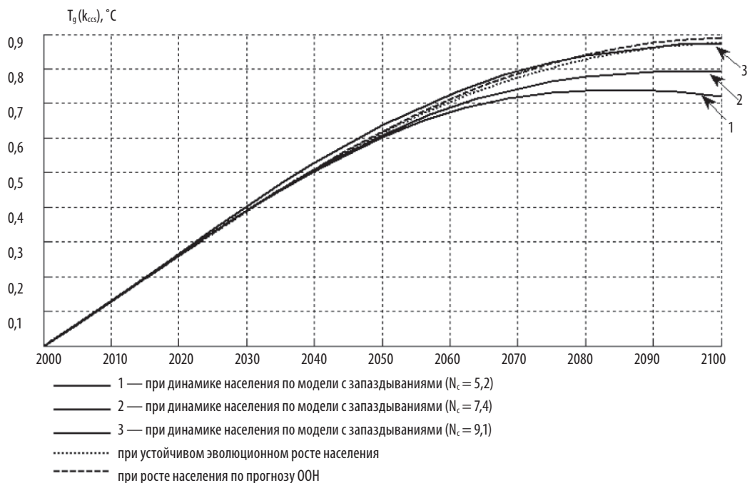
Рисунок 17. Отклонения средней глобальной температуры у поверхности Земли в XXI в. от значения в 2000 г. при использовании технологии CCS для улавливания и захоронения части \text{CO}_2
