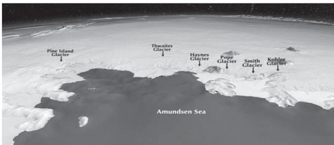
Рисунок 12. Таяние ледников и выбросы метана в Антарктиде
