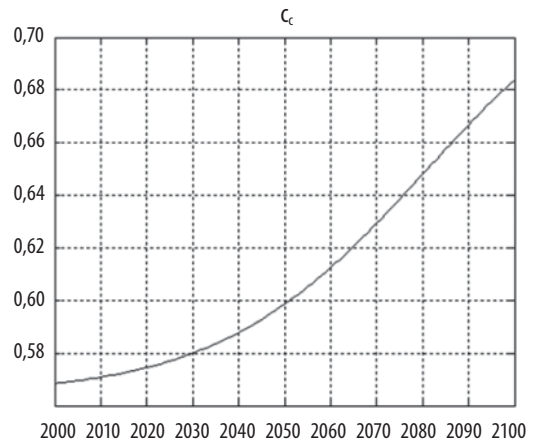
Рисунок 11. Среднемировой коэффициент углеродной интенсивности C_c
