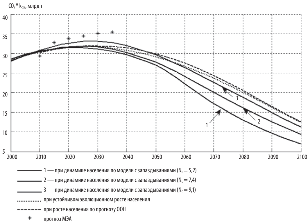
Рисунок 13. Динамика промышленных выбросов CO_2 в XXI в. (млрд т) при использовании технологии CCS для улавливания и захоронения части CO_2
