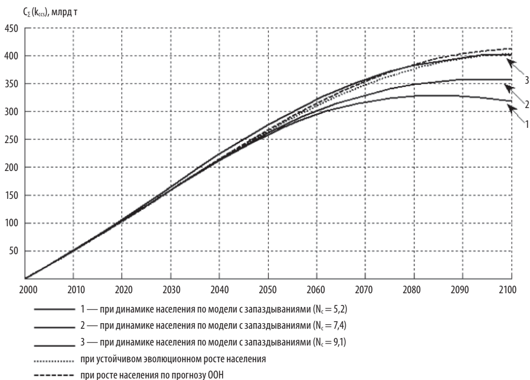
Рисунок 15. Динамика накопления углерода в атмосфере в XXI в. при использовании технологии CCS для улавливания и захоронения части CO_2
