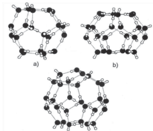
Рисунок 10. Структуры различных ассоциатов (кластеров) воды
